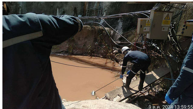
ตัวอย่างการติดตามตรวจสอบคุณภาพน้ำทิ้งอุโมงค์ - โครงการก่อสร้างทางรถไฟสายเด่นชัย-เชียงราย-เชียงของ (สัญญาที่ 2 ช่วงงาว-เชียงราย)
